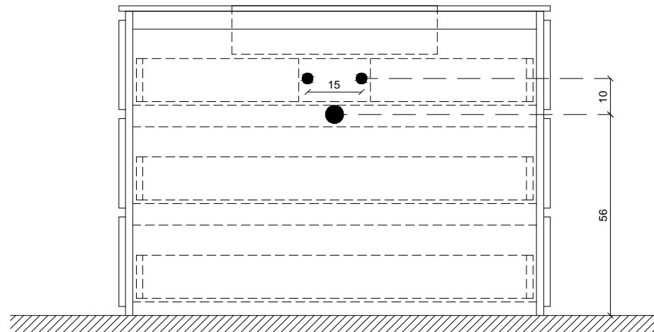
Prospetto / EVO_14
