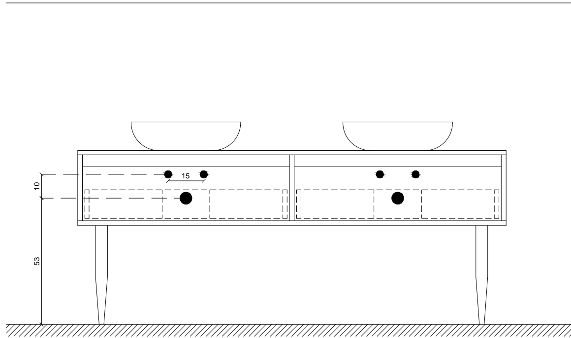
Prospetto / EVO_08
