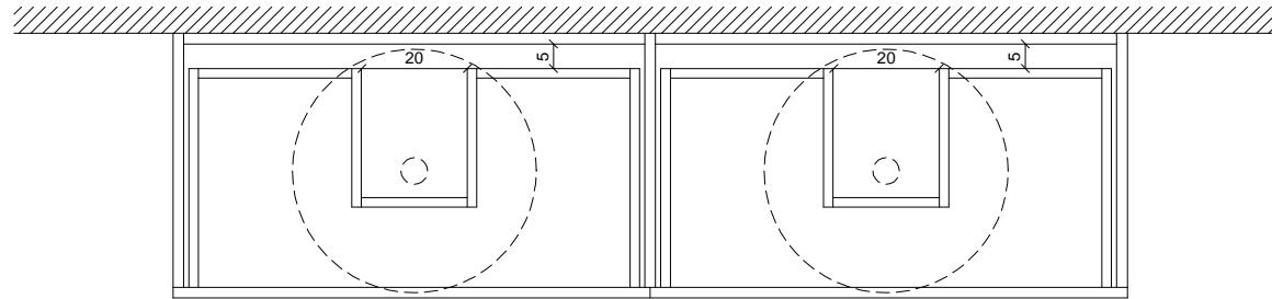
Pianta / EVO_08
