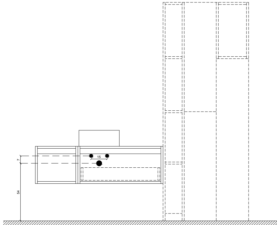
Prospetto / EVO_02
