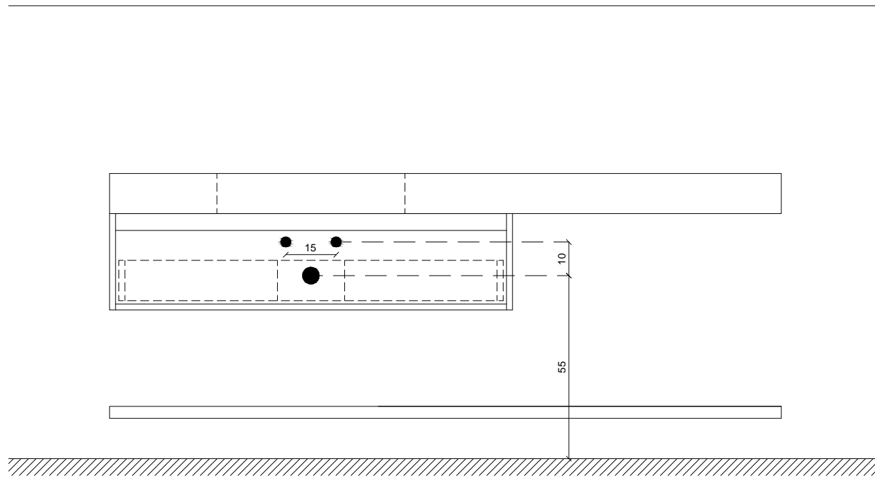
Prospetto / EVO_01
