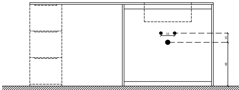
Prospetto / EVO Laundry_03
