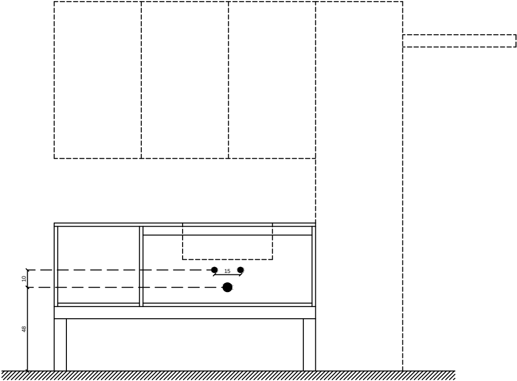
Prospetto / EVO Laundry_02
