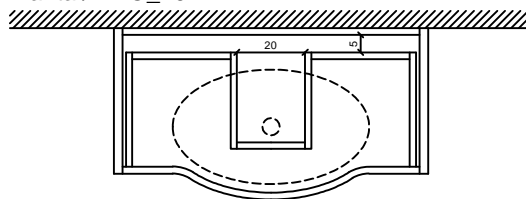
Pianta / EVO_16
