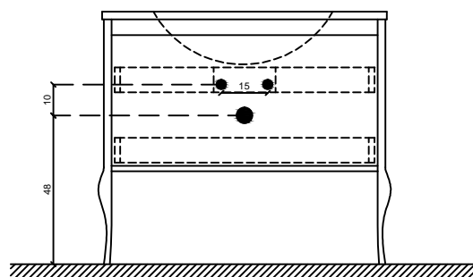
Prospetto / EVO_16
