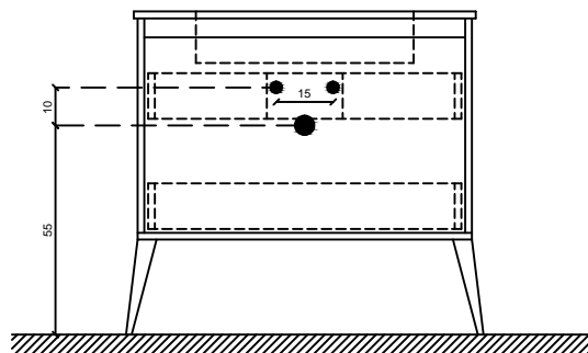
Prospetto / EVO_12
