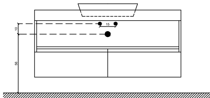
Prospetto / EVO_10
