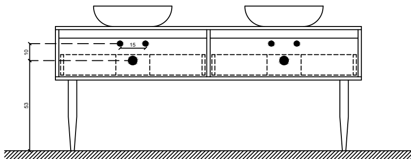
Prospetto / EVO_08
