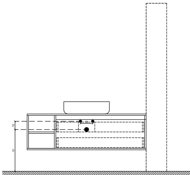
Prospetto / EVO_07
