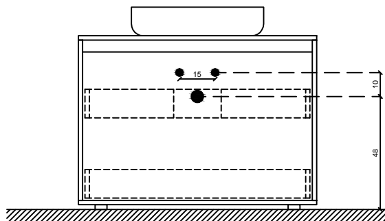
Prospetto / EVO_05
