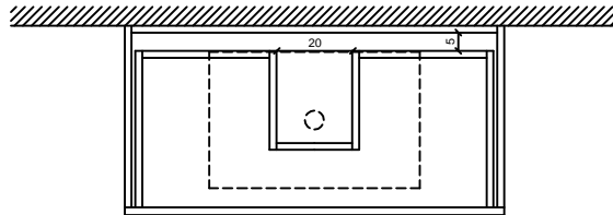
Pianta / EVO_05
