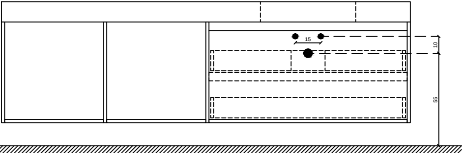
Prospetto / EVO_03
